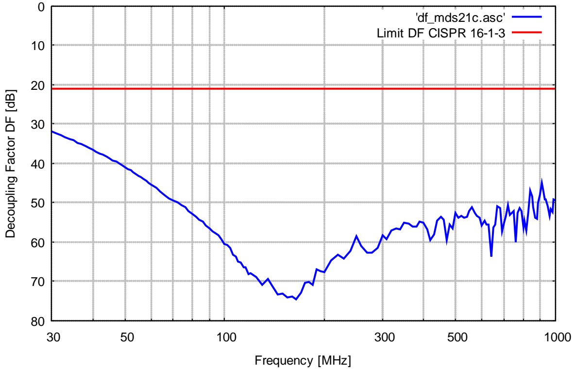
Entkopplungsmaß DF Decoupling Factor DF
