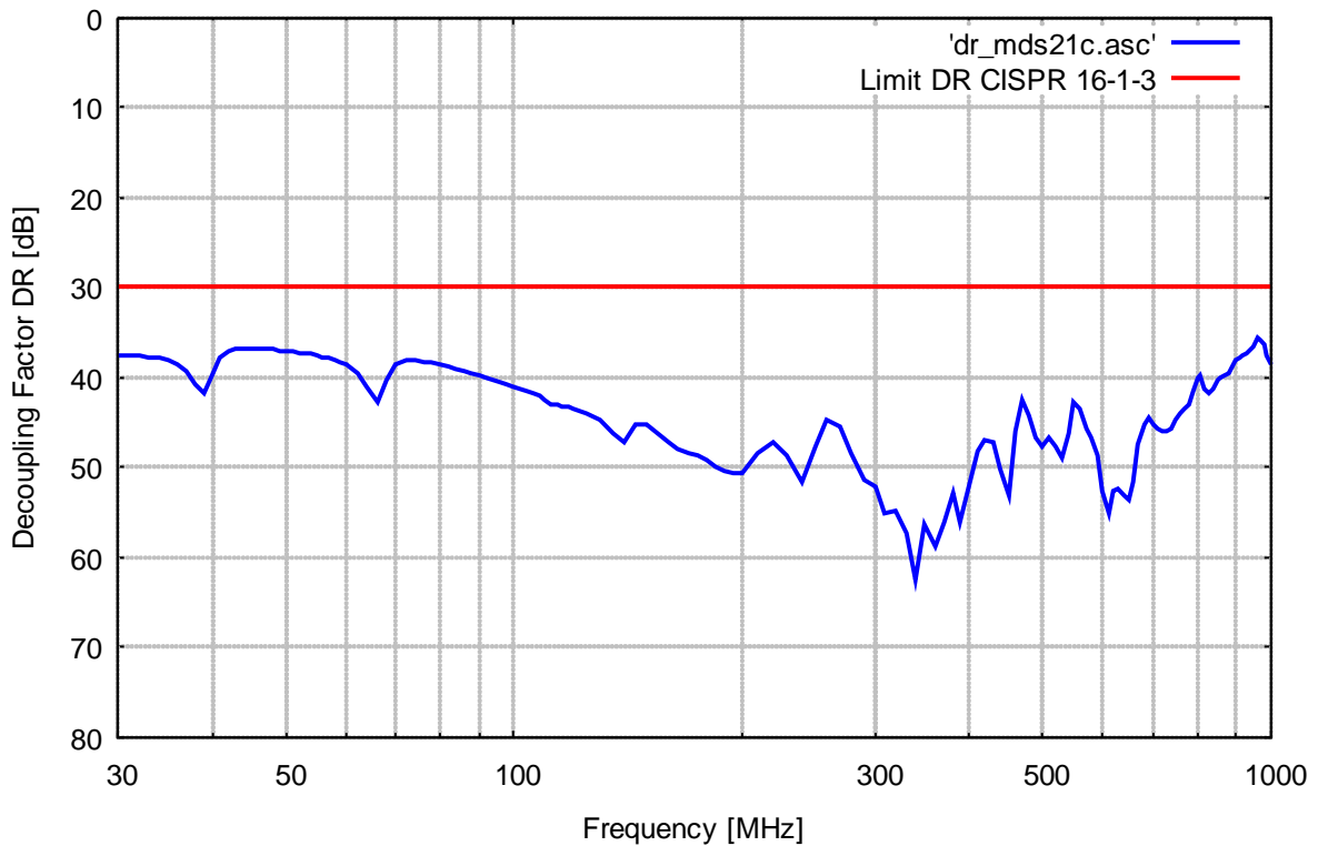
Entkopplungsmaß DR Decoupling Factor DR
